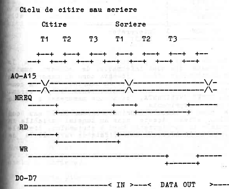
Fig. 4.2 Forme de unda pentru cicluri CPU
